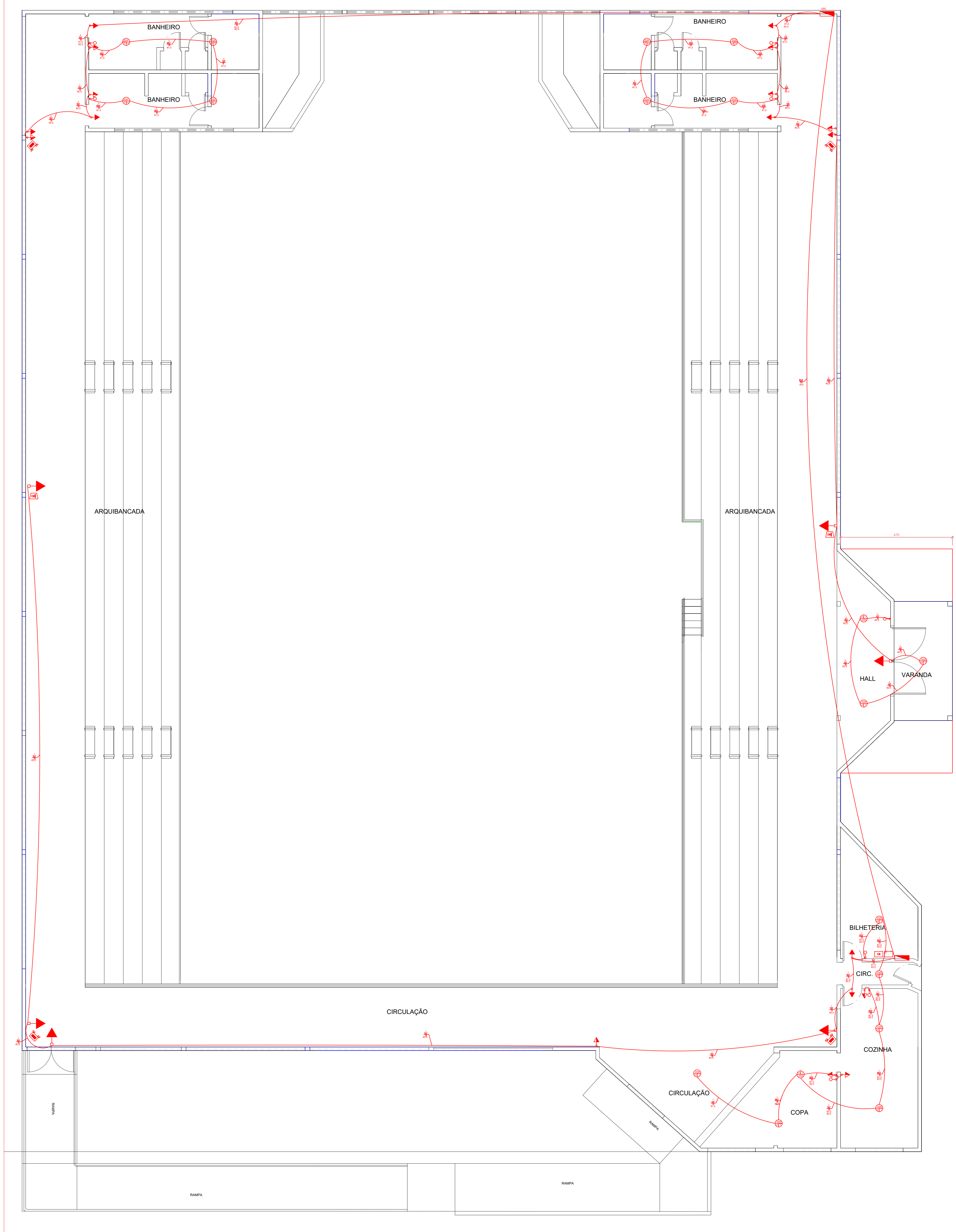
PLANTA BAIXA PAVIMENTO TÉRREO ESCALA 1:75
