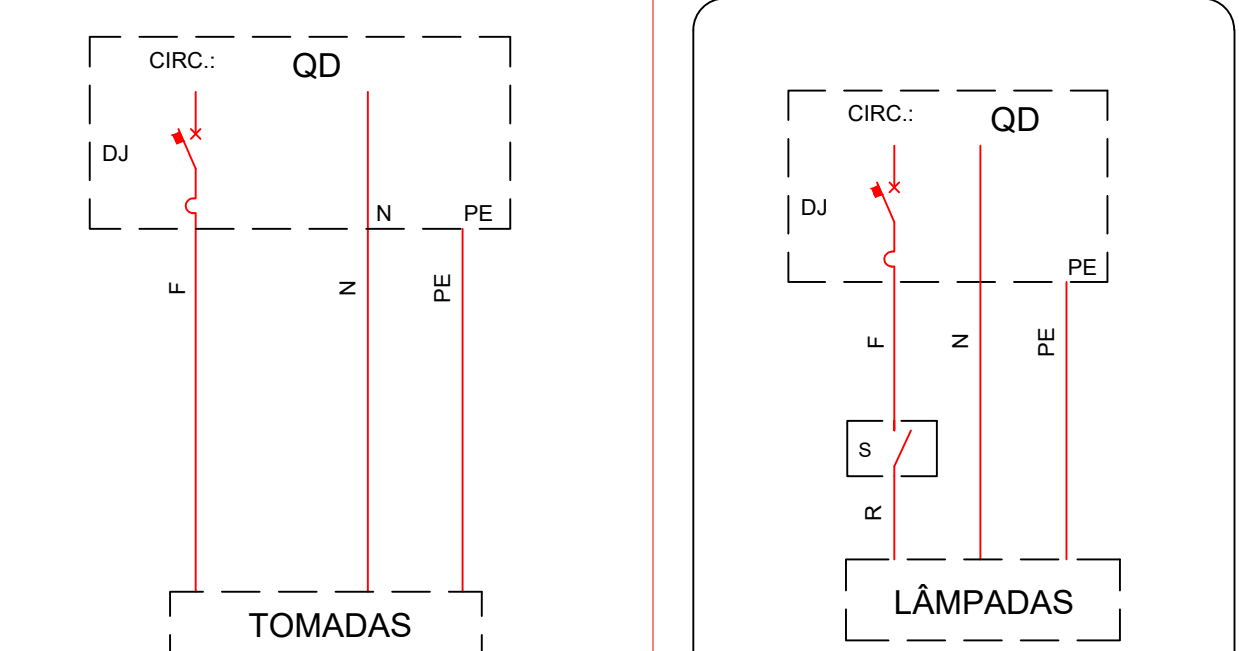
- TOMADA SIMPLES ATERRADA (2P+T) - INTERRUPTOR SIMPLES
