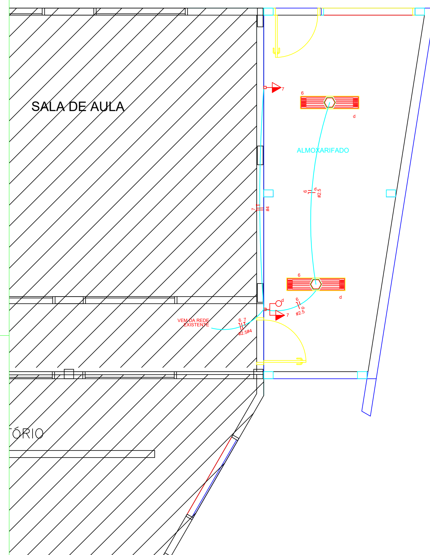
PLANTA BAIXA - ALMOXARIFADO ESCALA 1/50
