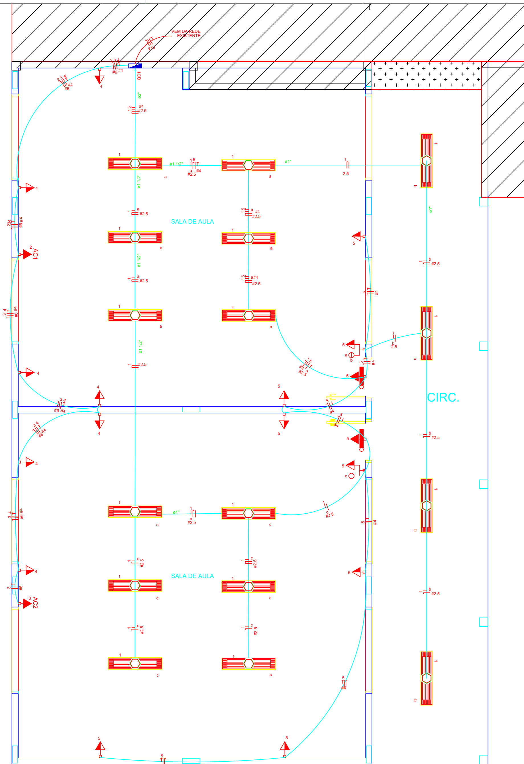
PLANTA BAIXA - SALA ESCALA 1/50
