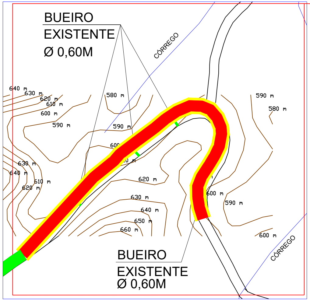
IPIRANGA TRECHO 024 PLANTA BAIXA ESC. 1:500
