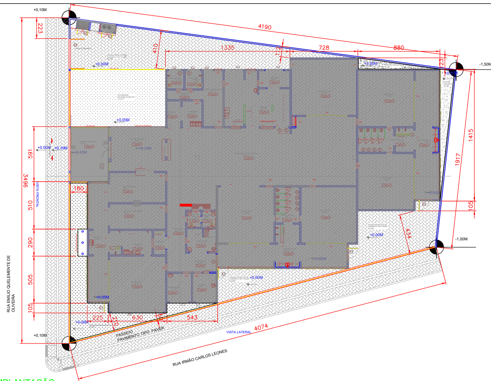
PLANTA DE IMPLANTAÇÃO ESCALA 1:200
