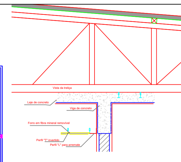
2 DETALHE 1: FORRO ESCALA 1/5
